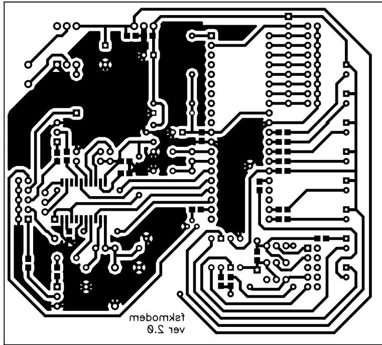
Проводники со сторона монтажа в зеркальном отображении
