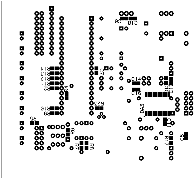
Сборочный чертеж, сторона монтажа
