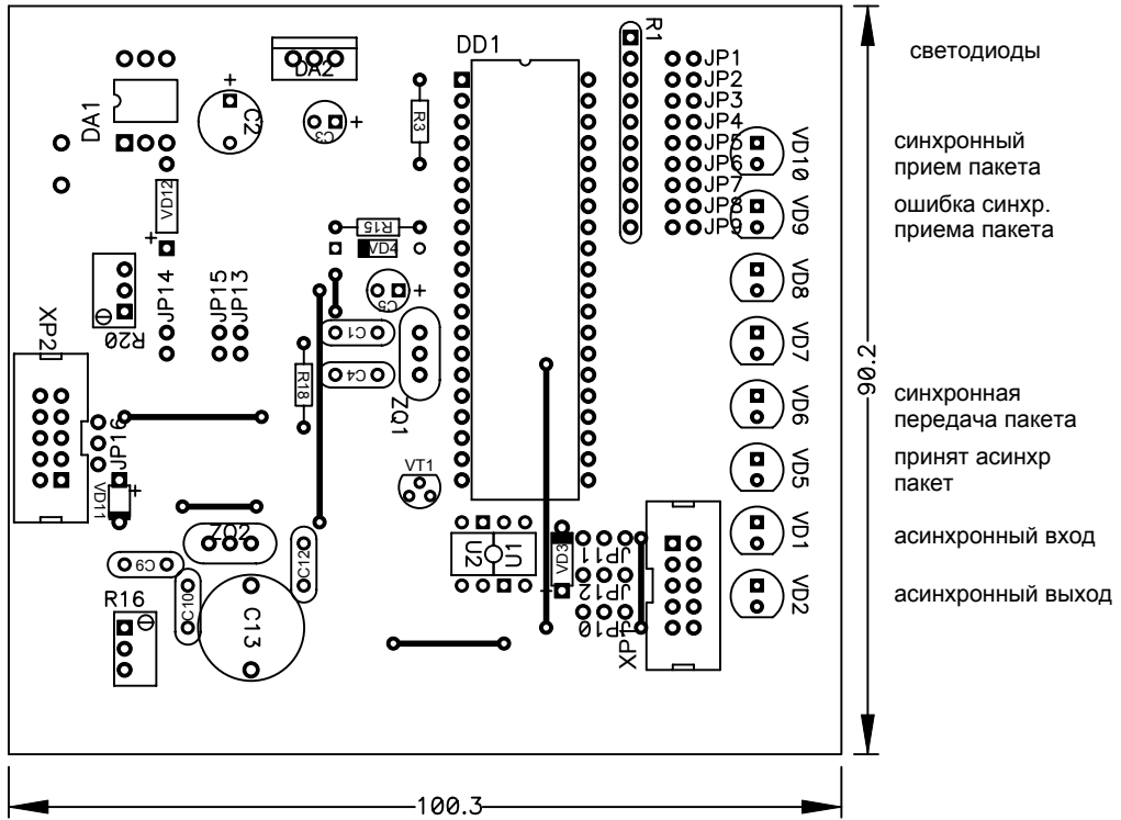
Сборочный чертеж, сторона компонентов
